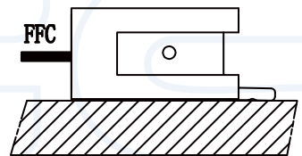
安装示意图 Assembly Layout
