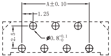
正针PCB寸法 PCB LAYOUT
