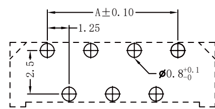
反针PCB寸法 PCB LAYOUT
