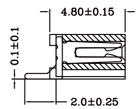
SEC: A-A
