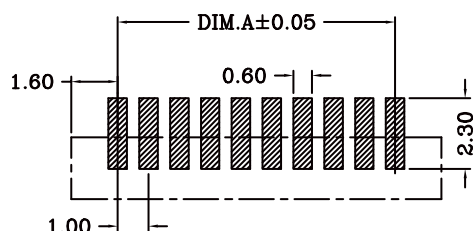
印制线路板 PCB P. C. B LAYOUT
