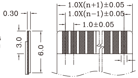
适用扁平电缆 (Proper cable)
