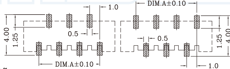
正针 PCB 寸法 Positive needle PCB LAYOUT 反针 PCB 寸法 Versa needle PCB LAYOUT
